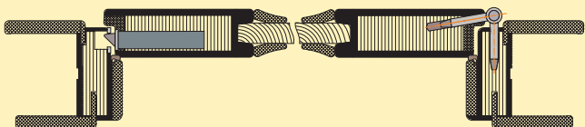
Сечение дверного блока линии 3000
